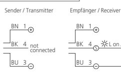
3-polig / 3-pin pnp
